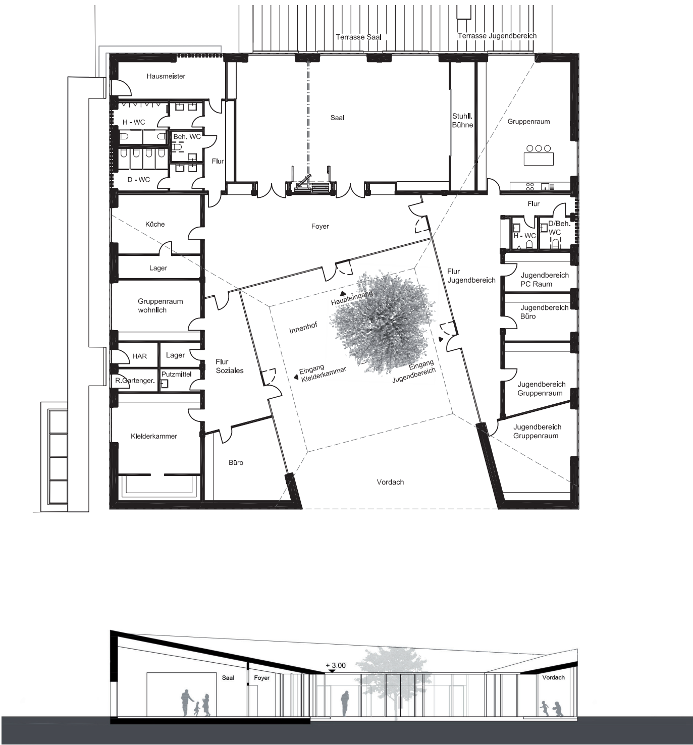
Grundriss und Schnitt
